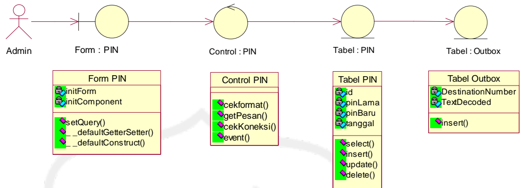
Gambar 3.20 Class Diagram Mengganti PIN
