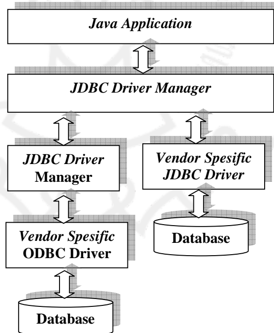
Gambar 2.1 Arsitektur JDBC
