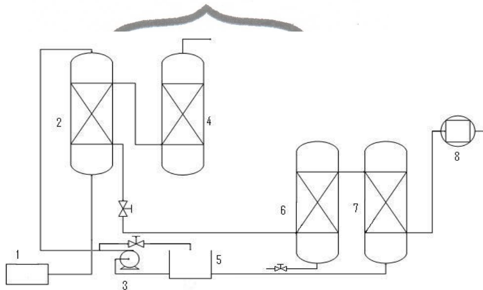
Gambar 3.4. Diagram alir proses pencucian biogas
