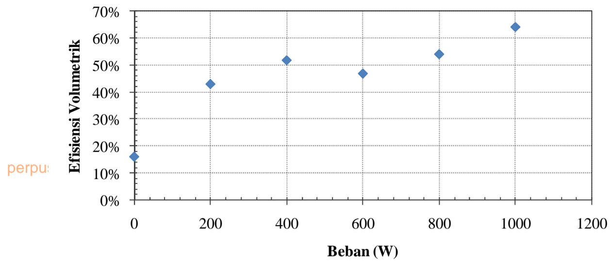
Gambar 4.2. Efisiensi volumetrik mesin berbahan bakar biogas.
