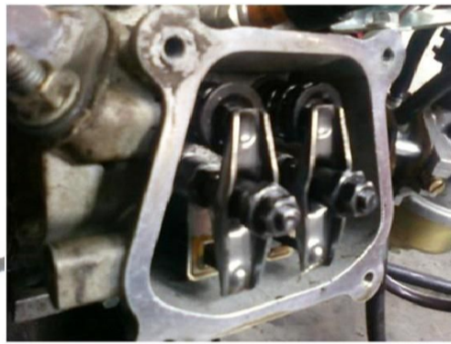
Gambar 3.5. Mekanisme Katup
