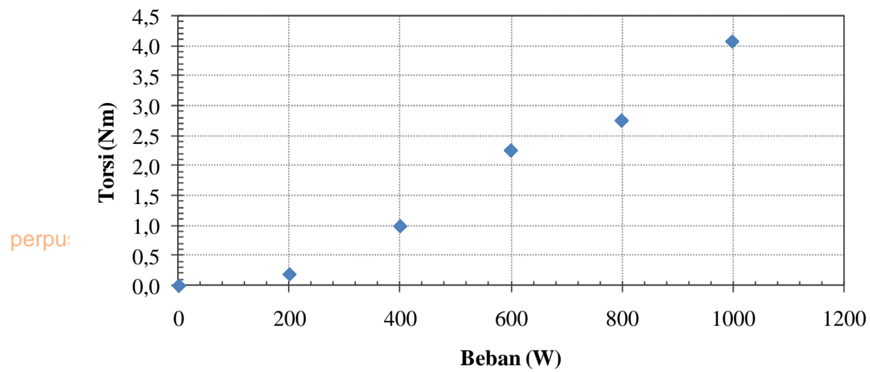
Gambar 4.1. Torsi mesin berbahan bakar biogas.
