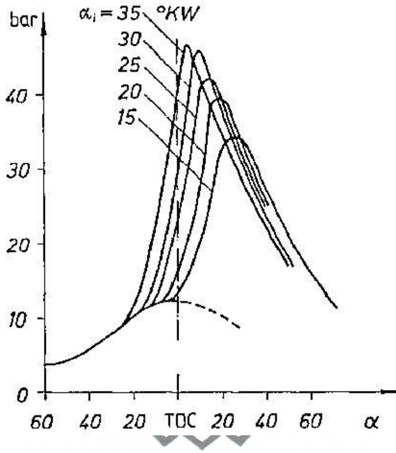
Gambar 2.4. Tekanan sebagai fungsi dari sudut pengapian (Mitzlatf, 1988).
