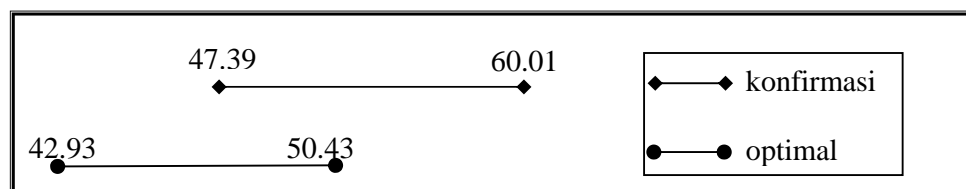
Gambar 4.5 Perbandingan nilai selang kepercayaan untuk rata-rata
