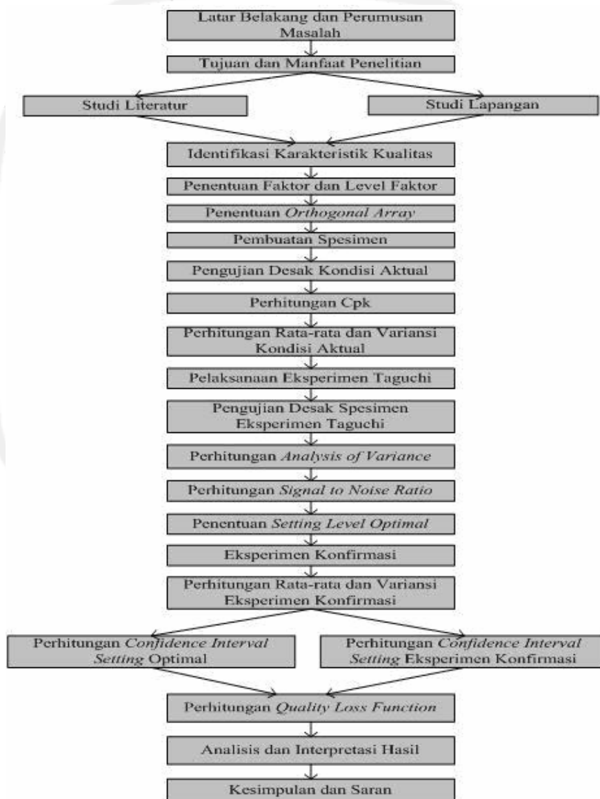
Gambar 3.1 Metodologi penelitian
