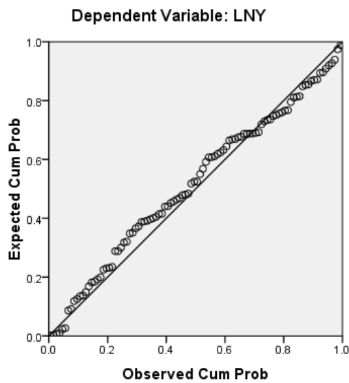
Gambar 5. P-Plot
